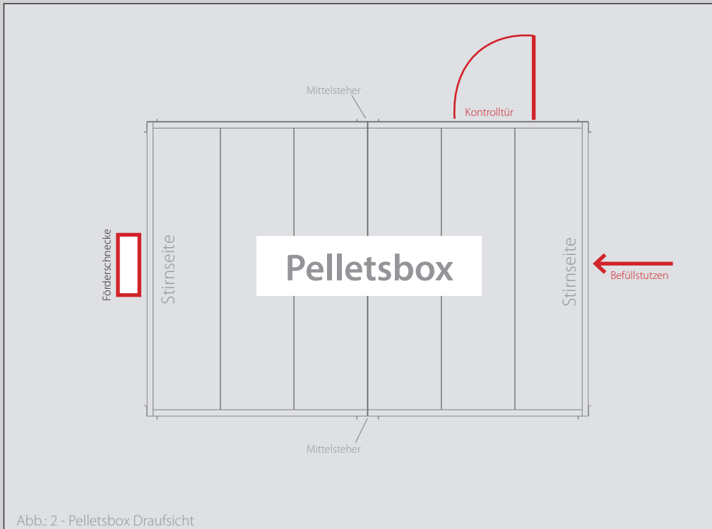
Abb.: 2 - Pelletsbox Draufsicht
